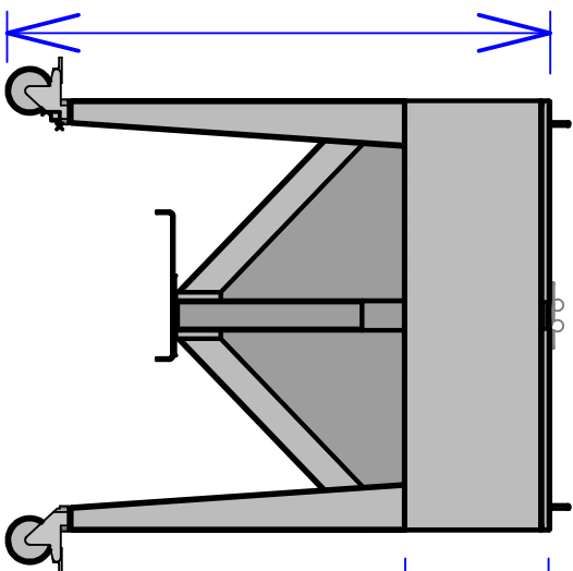
Vue auxiliaire
